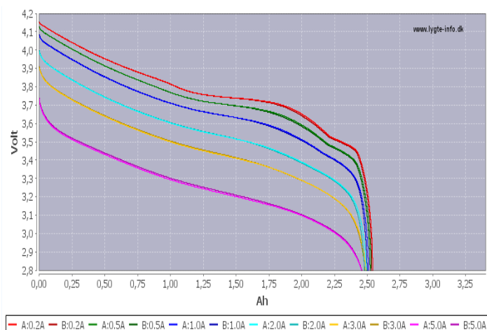
Charakterystyka rozładowania akumulatora XTAR 18650 2600mAh
