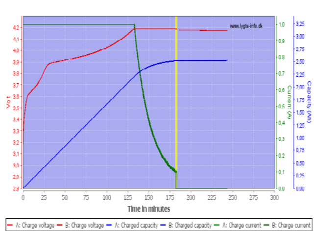
Charakterystyka ładowania akumulatora XTAR 18650 2600mAh
